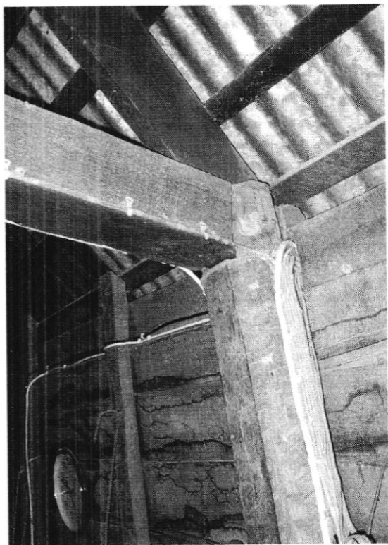
เห็นบากหูโป่ง (หูกะต่าย)
