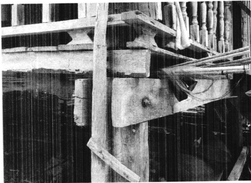
รายละเอียดจะเห็นการใช้ขางคู่ และ การใช้เสาเอียงค้ำทับหลังคาคลุม คันไถ
