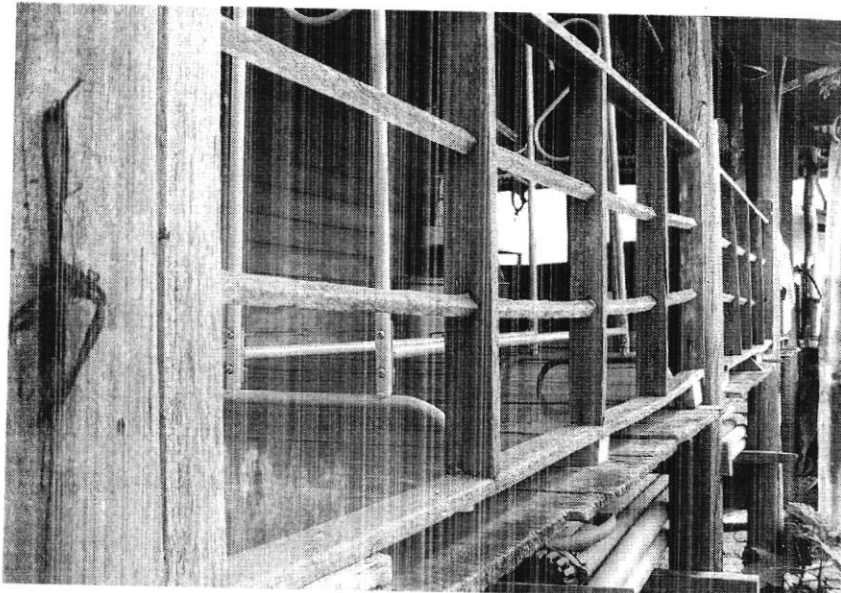
ราวระเบียงเจาะสอดไม้ ระเบียงสวยงาม
