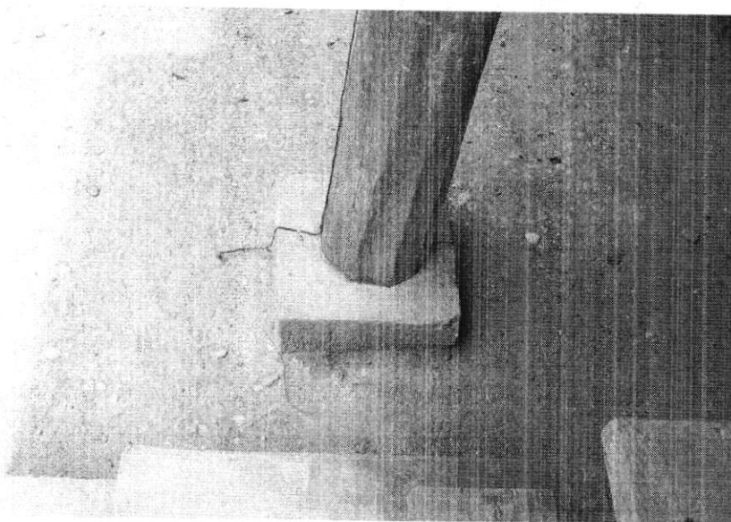
เสาและปูนรองพัวกันเสาผุ
