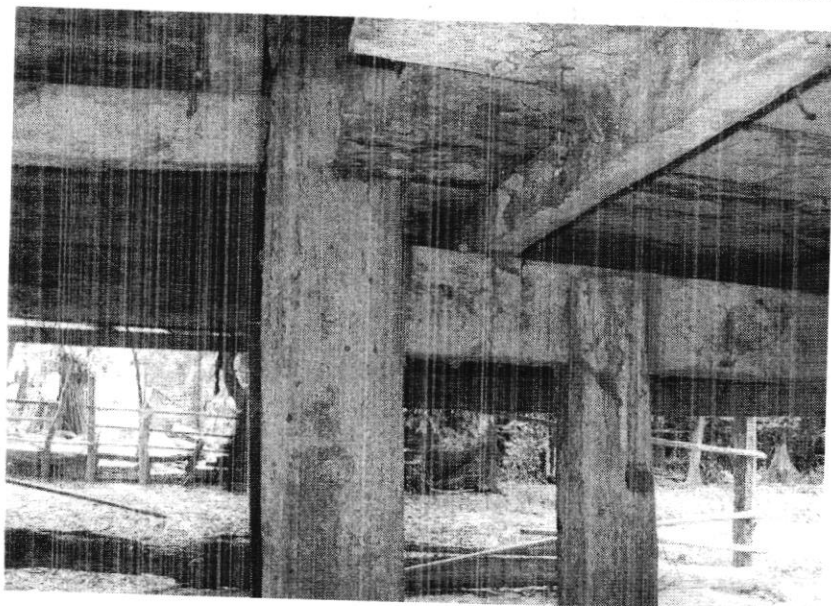
แสดงทางสอดเสา และเสารับ พื้นเขี้ยว
