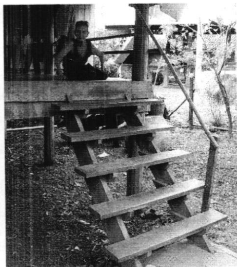
เรือนหัวลอยไทยกระเลิง หลังคาทรงปั้นหยา มีจั่วเล็ก ของนางประทุมวัลย์ บุษบา เลขที่บ้าน 1181 บ้านนามน อ.เมือง จ.นครพนม ฝาไม้แคน เสาไม้แต้ คานไม้แดง
