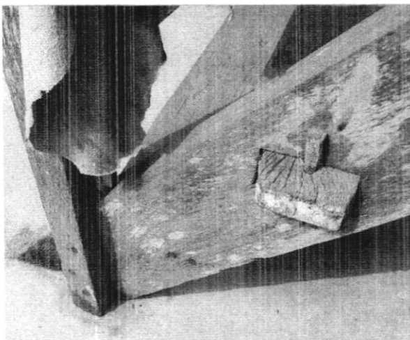
การเข้าเดือยแม่บันไดกับฐานนอน
