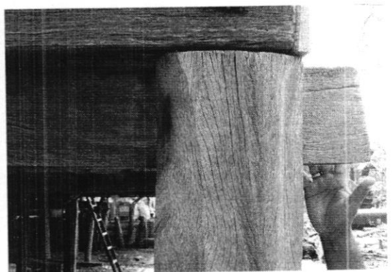
แบบหั่วเสาบานออก
