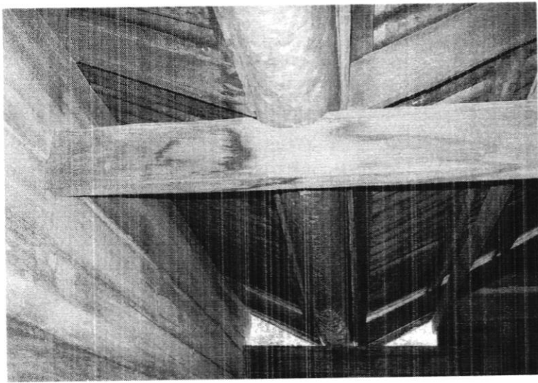
รางน้ำระหว่างหลังคา เรือน นอน และเรือนหัวถอย
