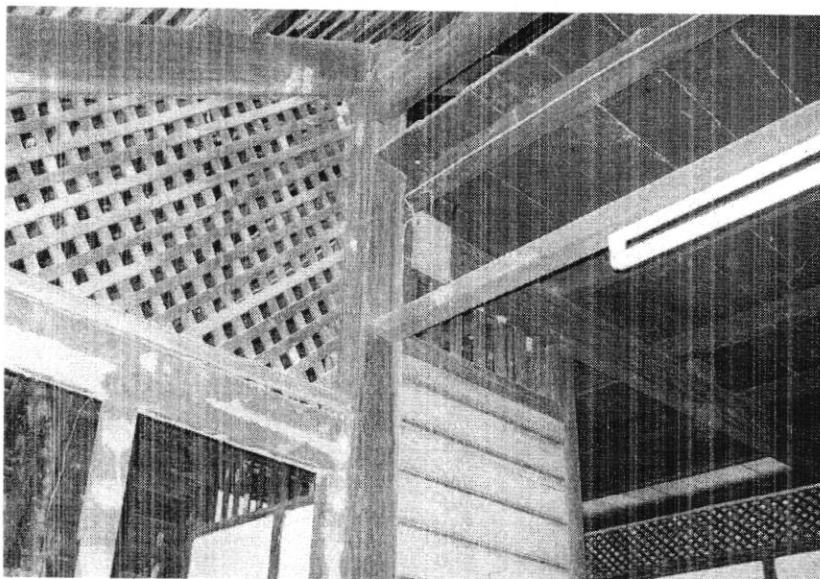
ช่องสามเหลี่ยมดีไม้ระแนงระบายลม เพดานเป็นที่เก็บของได้
