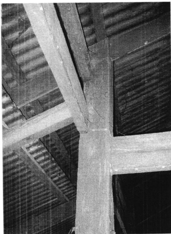
การยัด สยว, อะเส, ซื่อเข้ากับตัวเสาจะเห็นการลด ระดับซื่อกับเสา เพื่อให้อีกด้านใ้รางน้ำได้
