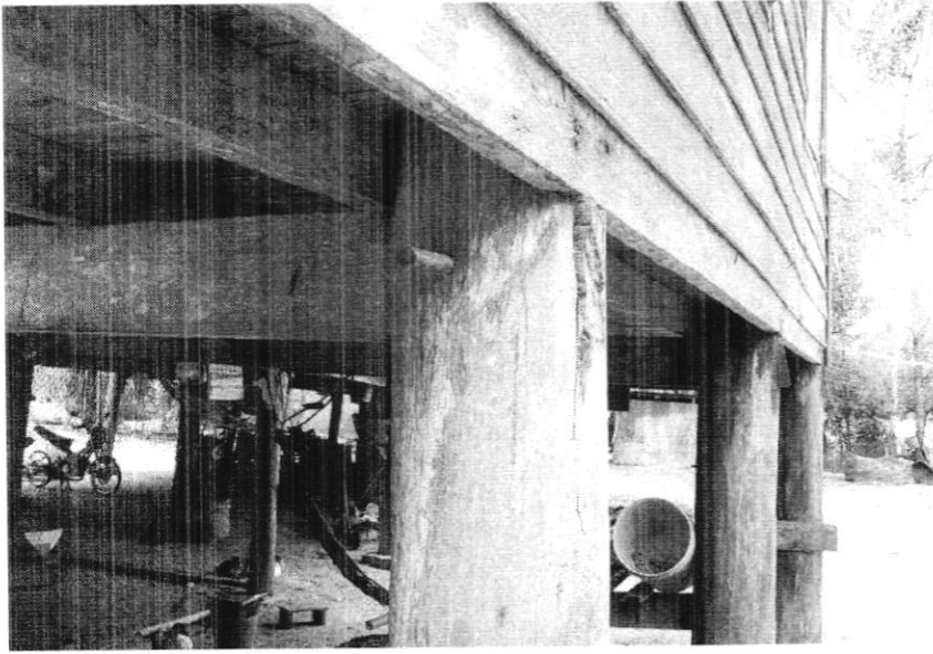
คานสอตกกลางเสา และเจาะรูใส่ เตี้ย (โร)
