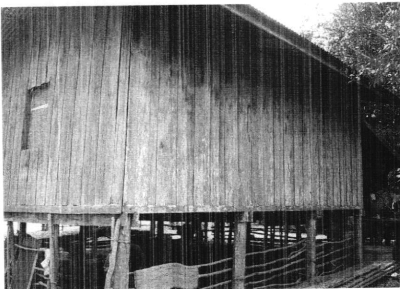
การตีฝาทางตั้ง
