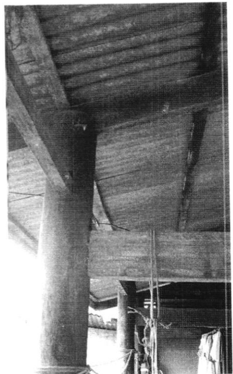
จันทัน (สยว) ผ่านกลางเสาพร้อมไร และคานยัดเสียบเสา
