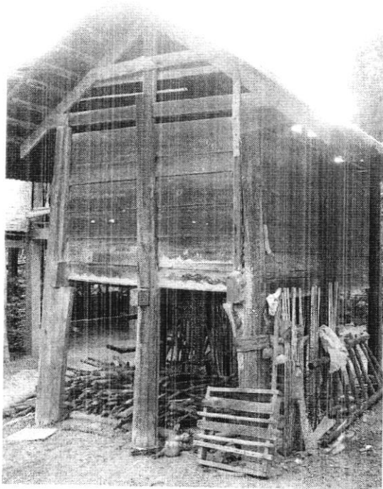
เจ้าข้าวไทยย้อ ตงขวาง บ้านเอื้อง อ.ศรีสงคราม
