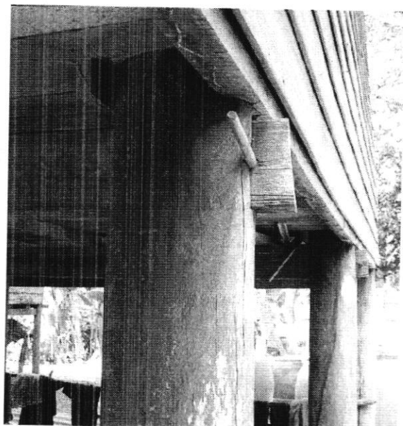
เสาและคานสอดพร้อมการยึดด้วยโร
