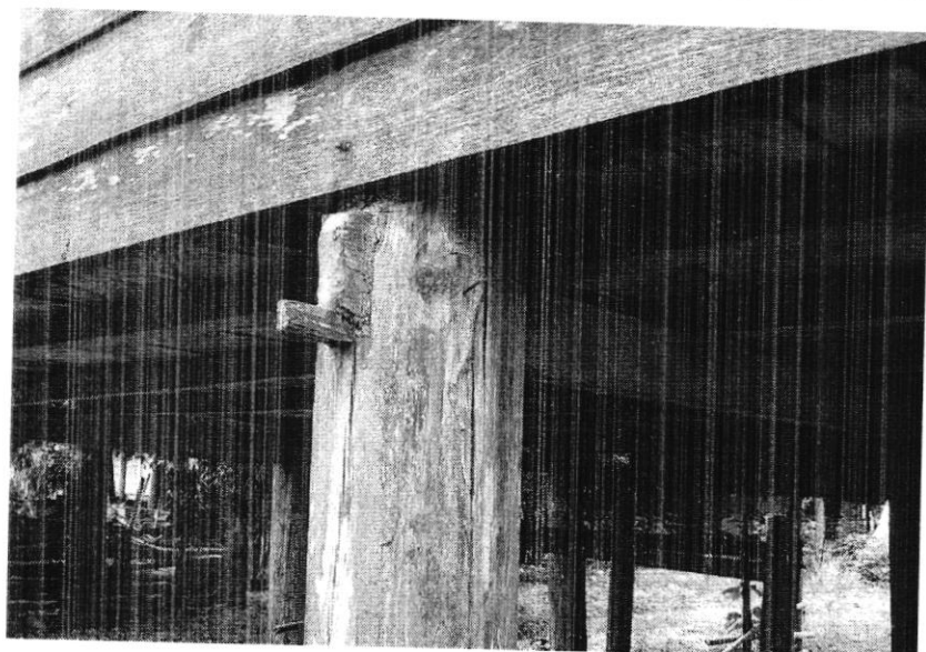
ลิ้มรองรับทางสอด
