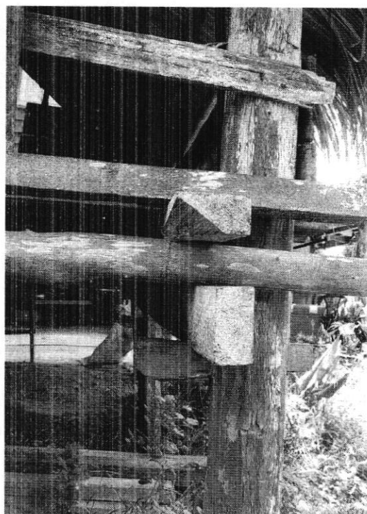
แสดงให้เห็นเตี้ย (ปิง) รับคานกลม และคานเหลี่ยม
