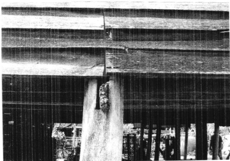
คานสอดกลางเสา
