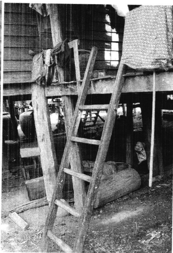
คันทันแบบโบราณ
