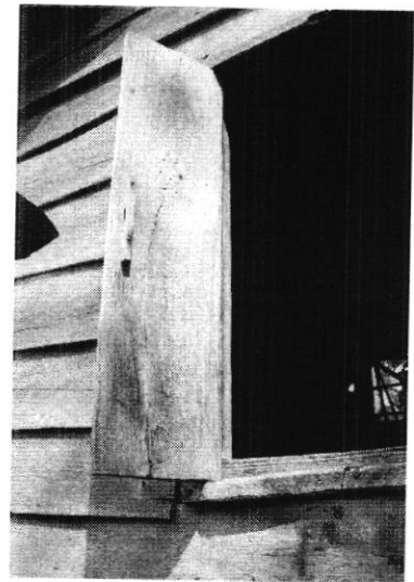
บานหน้าต่างใช้เดือย
