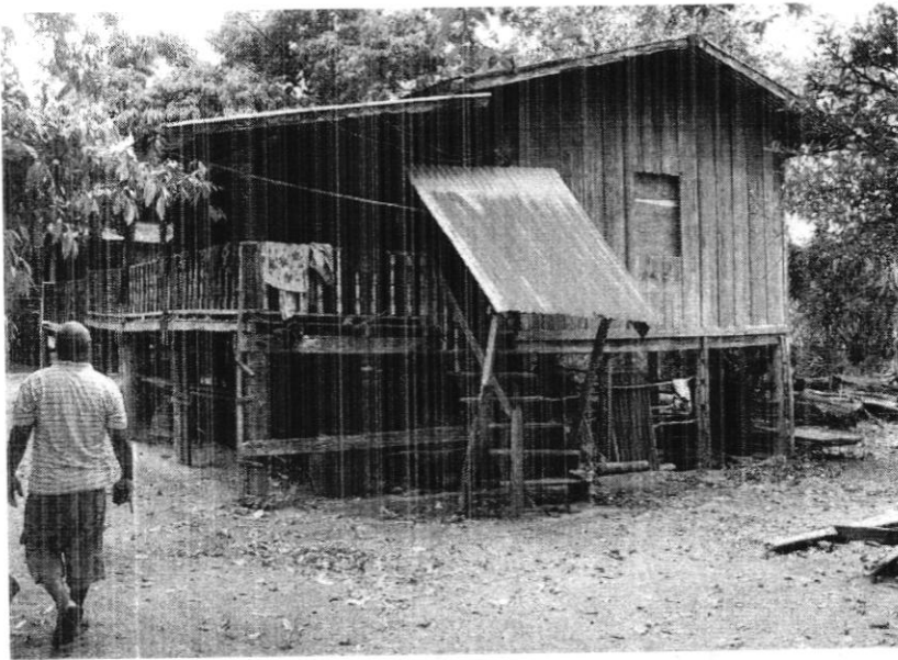
เรือนเกย (เตี้ย) กะเลิง ปากน้ำศรี สงคราม ไม้ไผ่บาก, ไม้ยาง ของพ่อสล่า บาศรีชาติ 37 หมู่ 12 วังโพธิ์ ต.ไชยบุรี อ.ท่าอุเทน อายุ 50 ปีขึ้นไป
