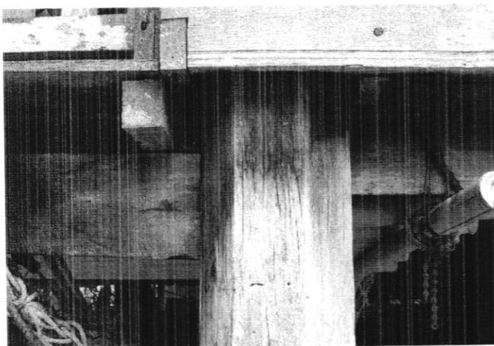
เสา 8 เหลี่ยมพร้อม ขาง (คาน) สอด
