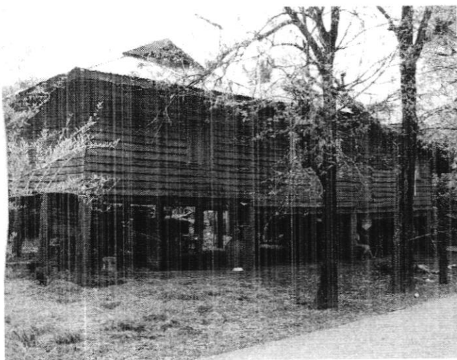
เรือนหัวลอยไทยกระเลิง หลังคาทรงปั้นหยา มีจั่วเล็ก ของนางประทุมวัลย์ บุษบา เลขที่บ้าน 1181 บ้านนามน อ.เมือง จ.นครพนม ฝาไม้แคน เสาไม้แต้ คานไม้แดง
