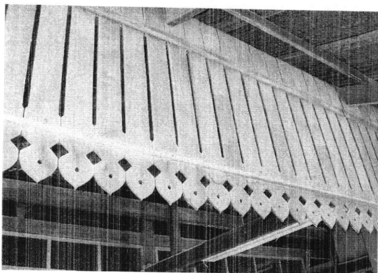
ผนังด้านหน้าเรือนหัวลอย จะมีผนังตกแต่งเป็นลายซ้อย สวยงาม
