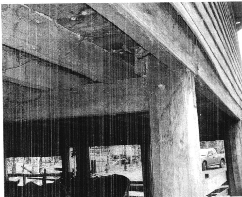
พื้น, ตง, ขางสอ, เสากลม
