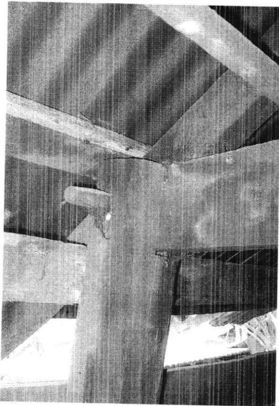
บากหูกกระต่าย พร้อมการตอกโร
