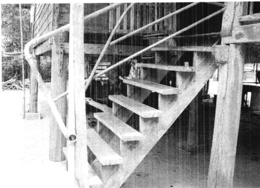
บันไดด้านข้าง
