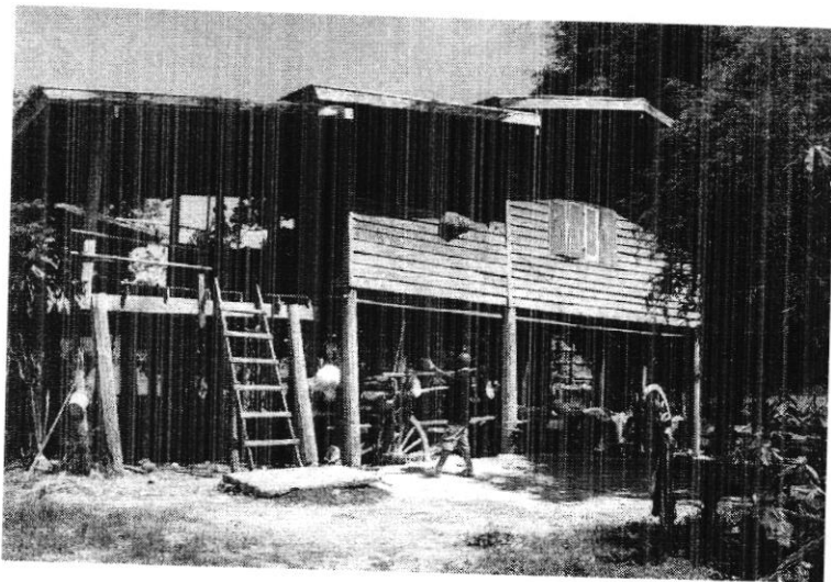
เรือนไทยชำ เจ้าของ นางบัวลย คำมุงคุณ 81 หมู่ 2 บ้านโสกแมว ต.อุ้มเหมา อ.ธาตุพนม
