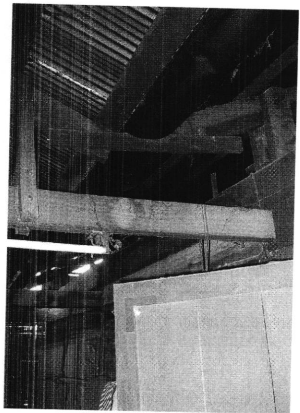
การต่อเชื่อมกับจันทันนอกเสาจะเห็นการบาก (หุ กระต่าย) ยึดด้วยไผ่
