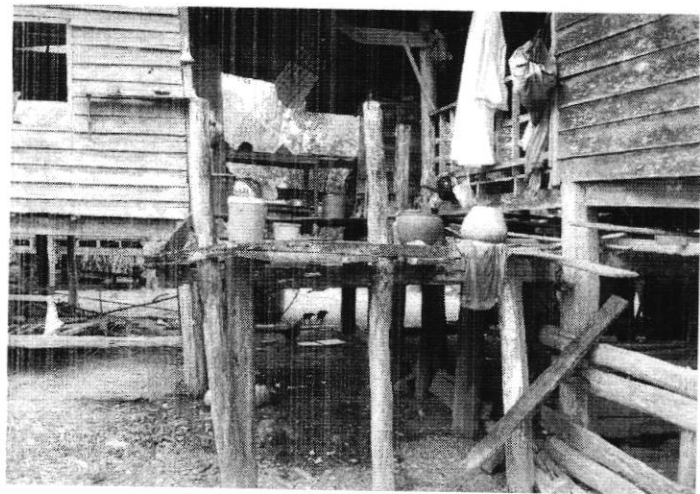
เรือนครวัดตรงหน้าจั่ว (สีหน้า) จะโล่ง ให้แสงและควันระบาย
