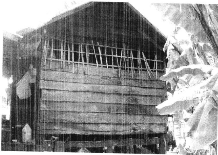
ช่องคอสองของเรือนครัว ระบายควัน
