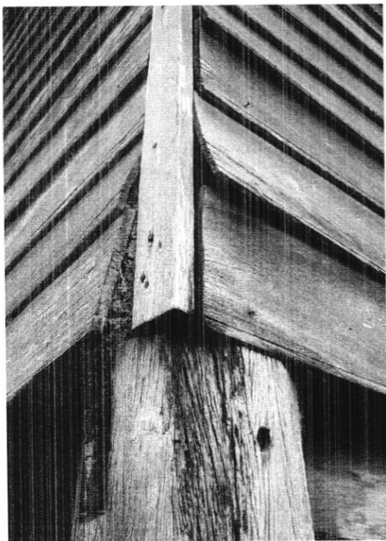
มุมอาหารเรือนนอนจะเห็นเสากลมและข้างสอ มีรอยัดไม่มีกะทอ (กรอบทอ)
