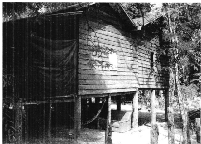
ด้านข้างเรือนจะเห็นการลดระดับพื้น จากคานสอดที่ลด ระดับ
