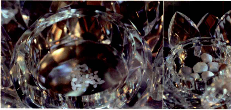
พระอัฐิธาตุหลวงปู่เสาร์ กนตสีโล ประดิษฐานที่วัดเลียบ
