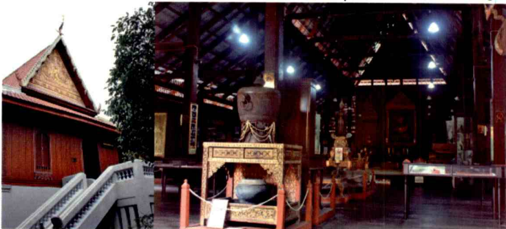
พิพิธภัณฑ์วัดศรีอุบลรัตนาราม
