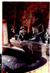
รอยพระพุทธรูปจำลองพระเจ้าองค์เงิน
