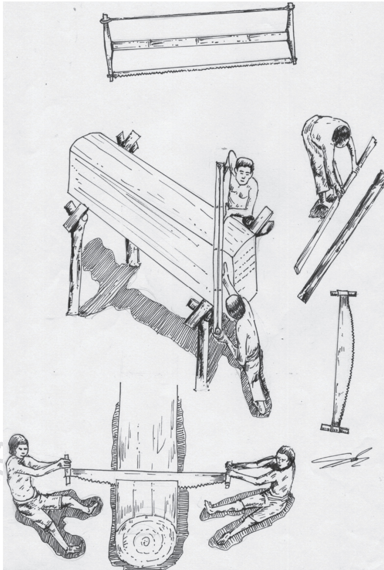
รูปที่ 3.26 เครื่องมือช่างไม้ (3)
