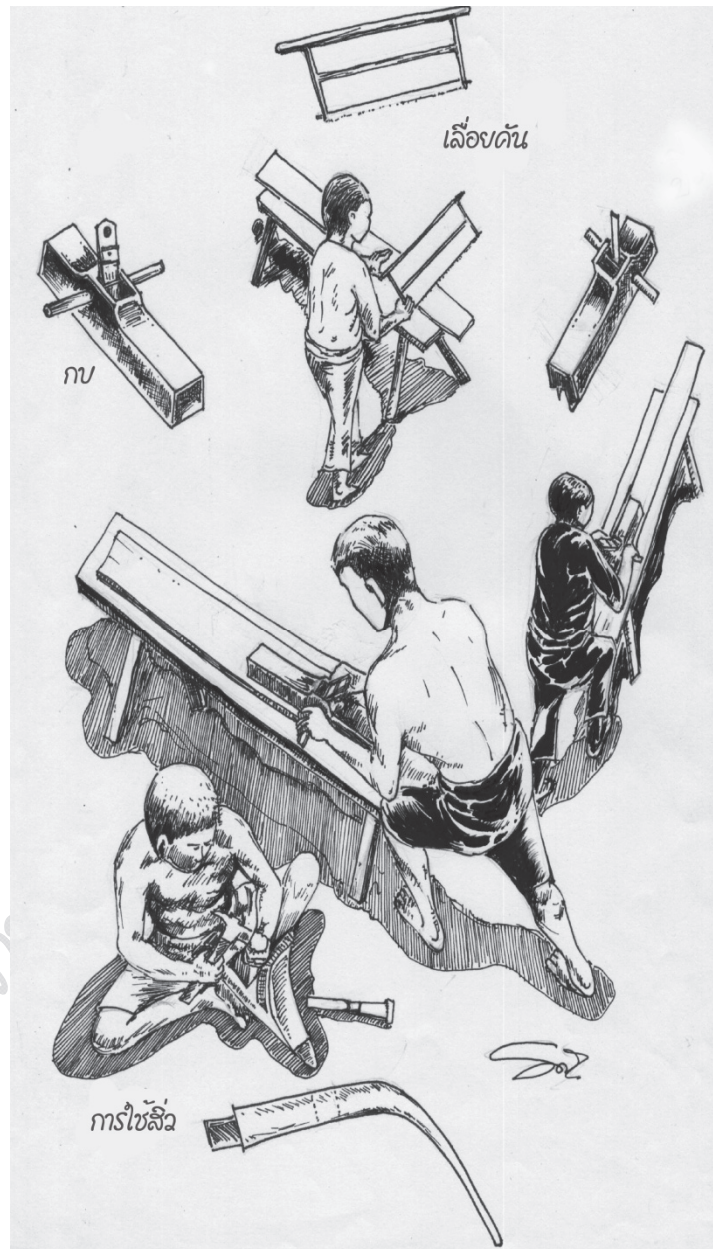
รูปที่ 3.25 เครื่องมือช่างไม้ (2)
