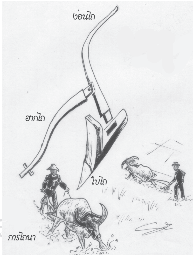
รูปที่ 3.29 ไถ (1)
